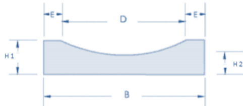
SEZIONE ELEMENTO CUNETTA
